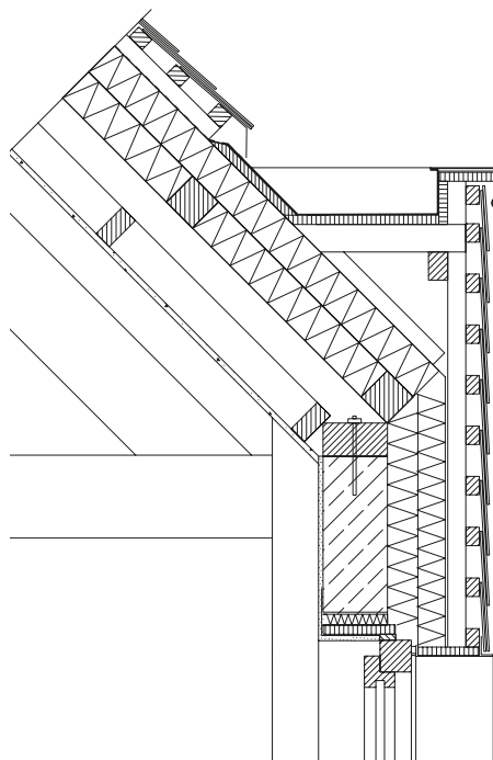
Bakgoot in combinatie met gevelbekleding met leien | verticale doorsnede
